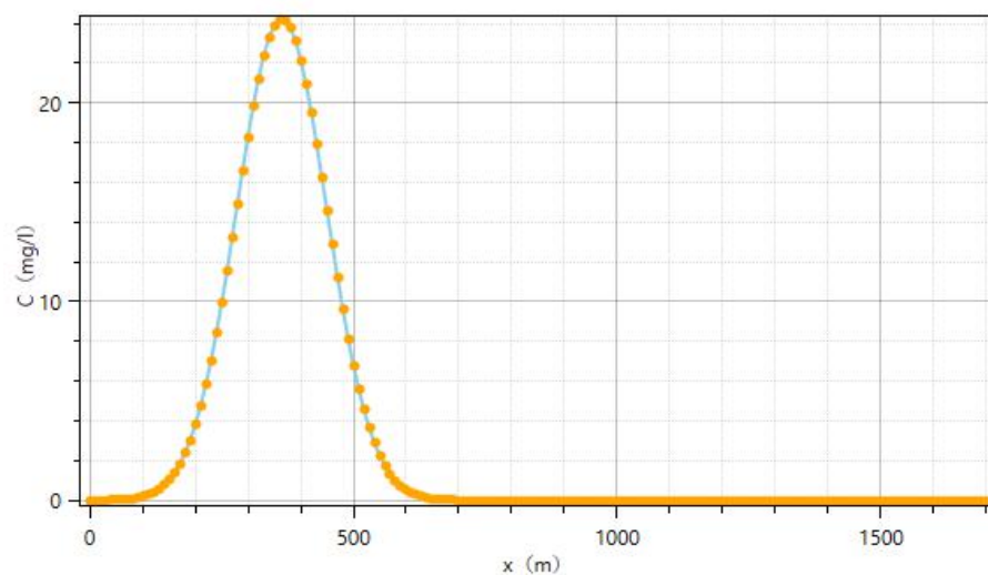
y=0, t=1000d 氨氮浓度变化曲线
