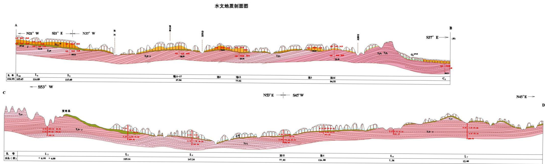
附图 5.6-2 项目所在区域水文地质剖面图
