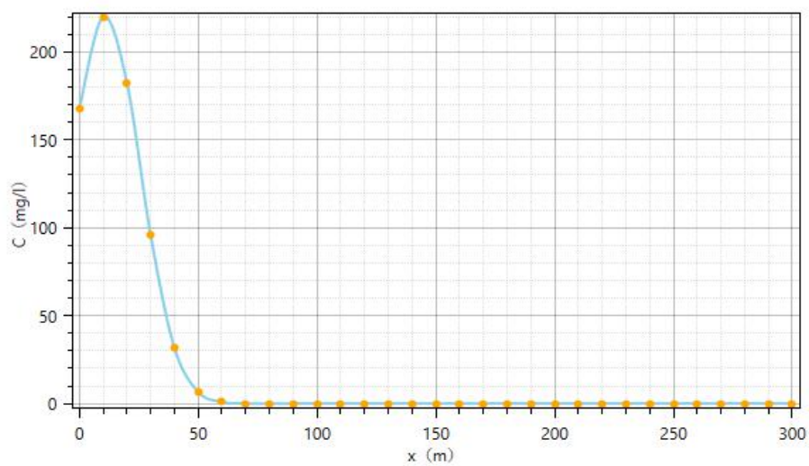
y=0, t=30d 硫酸盐浓度变化曲线
