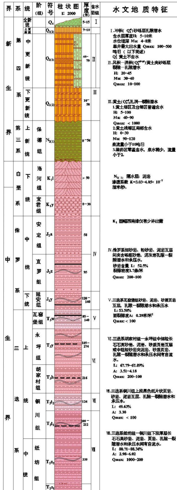
附图 5.6-3 区域综合水文地质柱状剖面图
