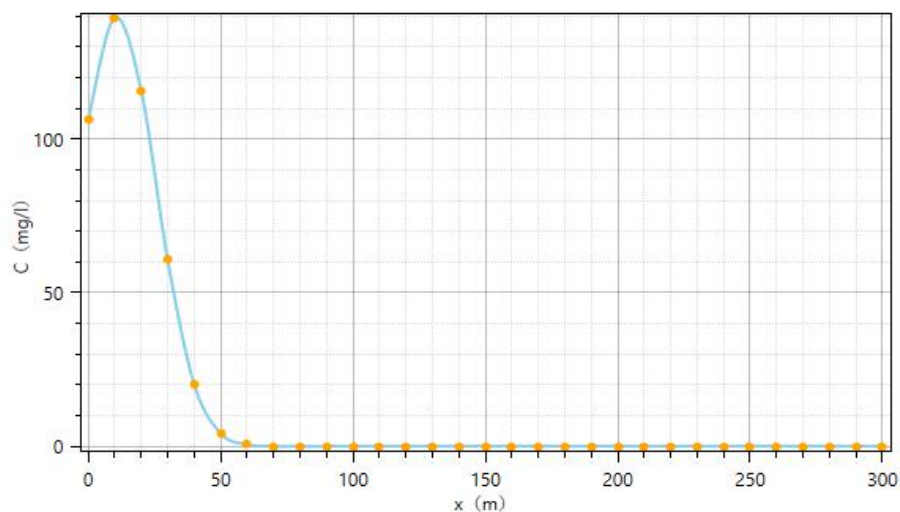
y=0, t=30d 氨氮浓度变化曲线
