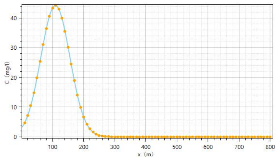
y=0, t=300d 氨氮浓度变化曲线
