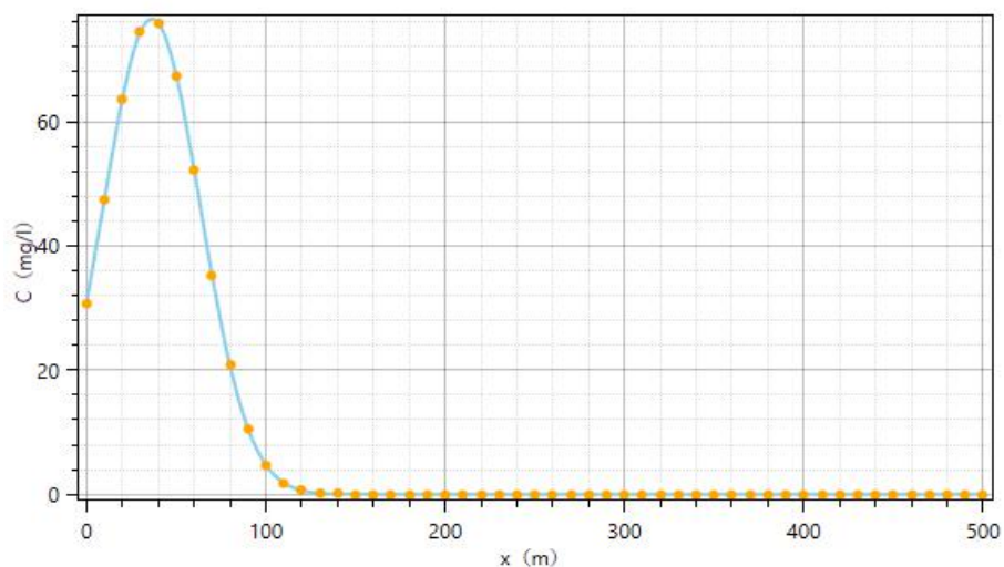
y=0, t=100d 氨氮浓度变化曲线
