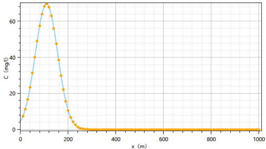
y=0, t=300d 硫酸盐浓度变化曲线
