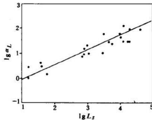
图5.6-1 孔隙介质数值模型的 \lg \alpha_L — \lg L_s 图
