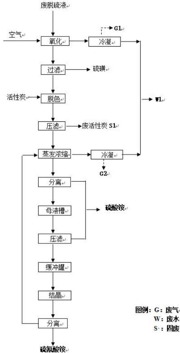
图 2.3-1 工艺流程图
