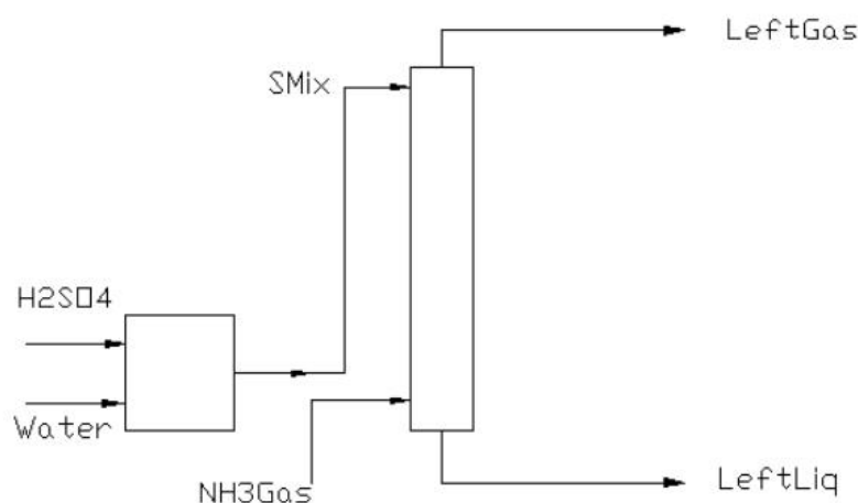
图 6.2-1 酸洗塔工作示意图
