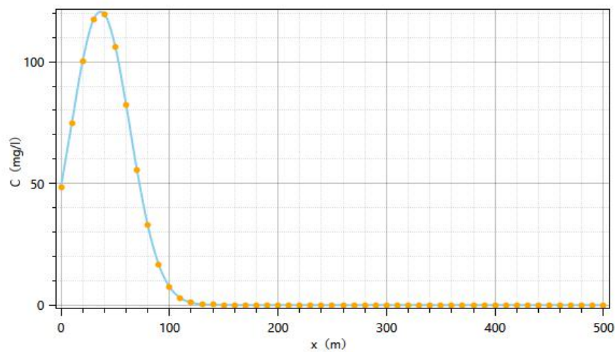
y=0, t=100d 硫酸盐浓度变化曲线
